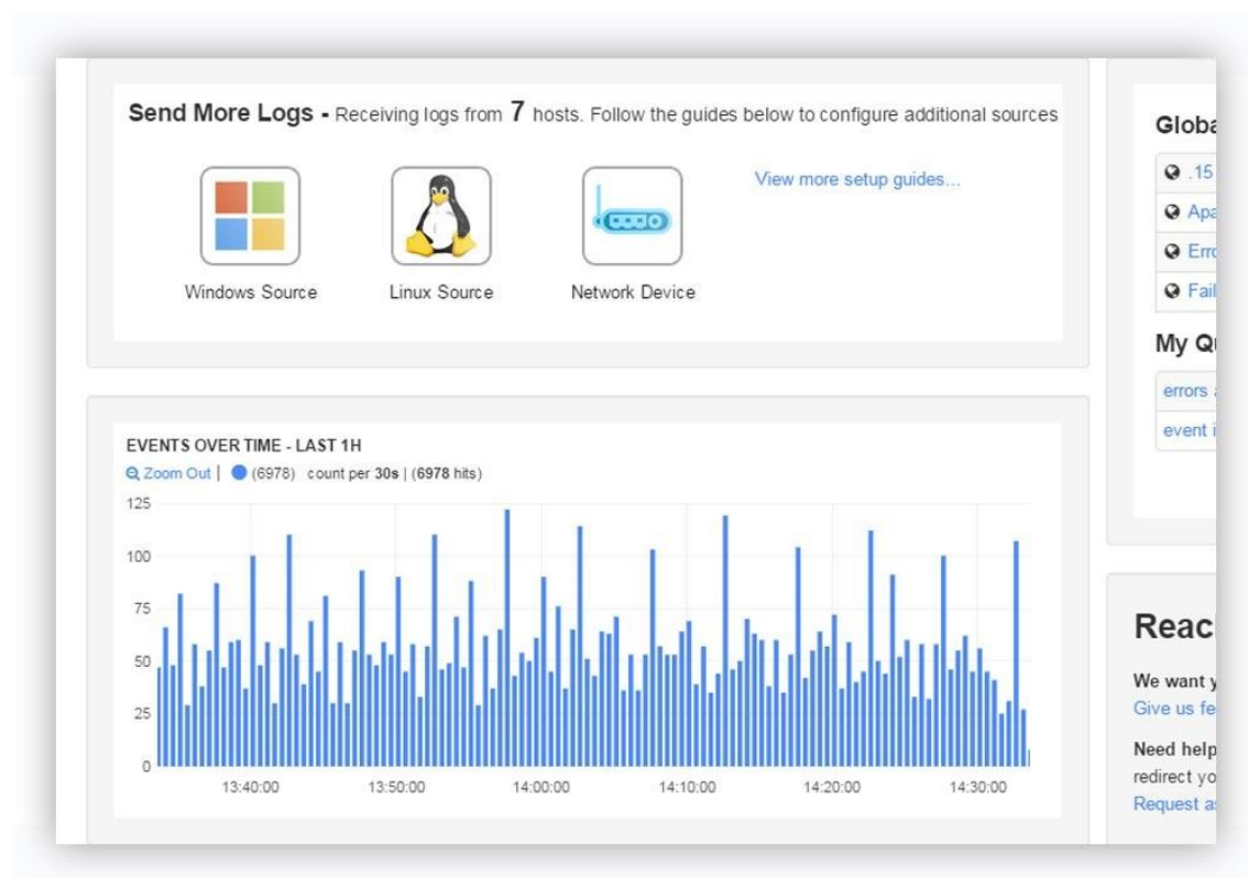
Figura 9 - Alta Escalabilidade
