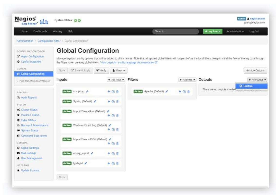
Figura 7 - Arquitetura Extensível
